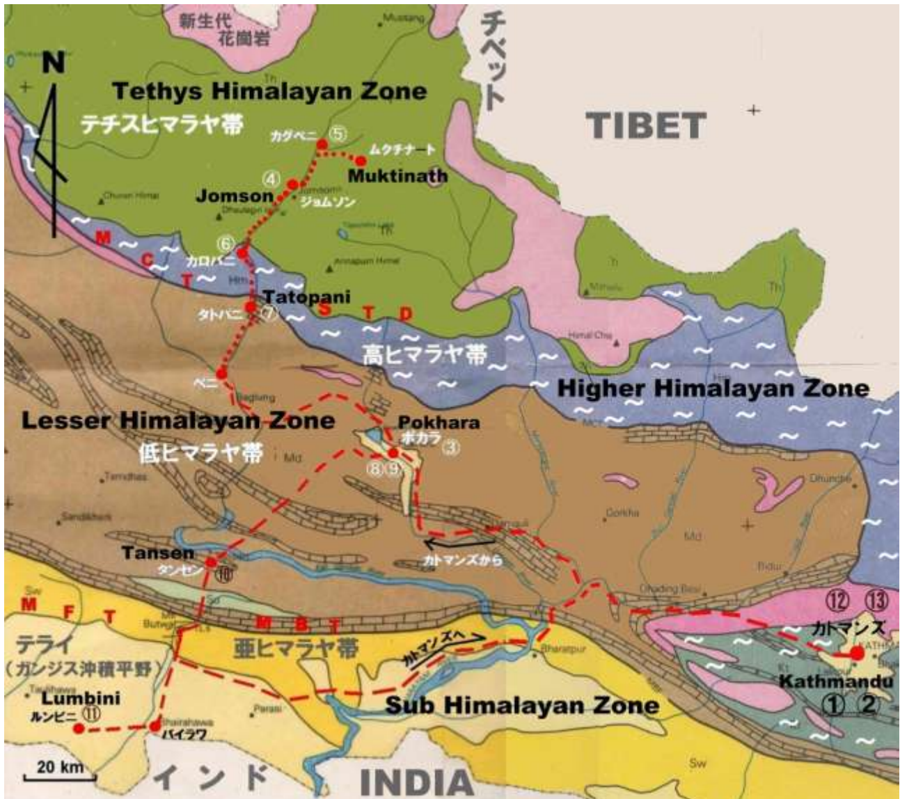
第6回学生のヒマラヤ野外実習ツアーのコースと日程(ベースの地質図はネパール地質鉱山局1981)MFT:主前縁衝上断層、MBT:主境界衝上断層、MCT:主中央衝上断層、STD:南チベットディタッチメント、赤点線(徒歩)と破線(車)は実習ルート、赤●は宿泊予定地、①~⑬は宿泊日程。
